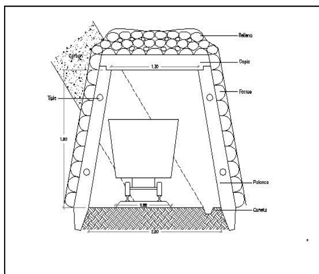
Figura 2: Esquema de una puerta alemana con sus componentes.
