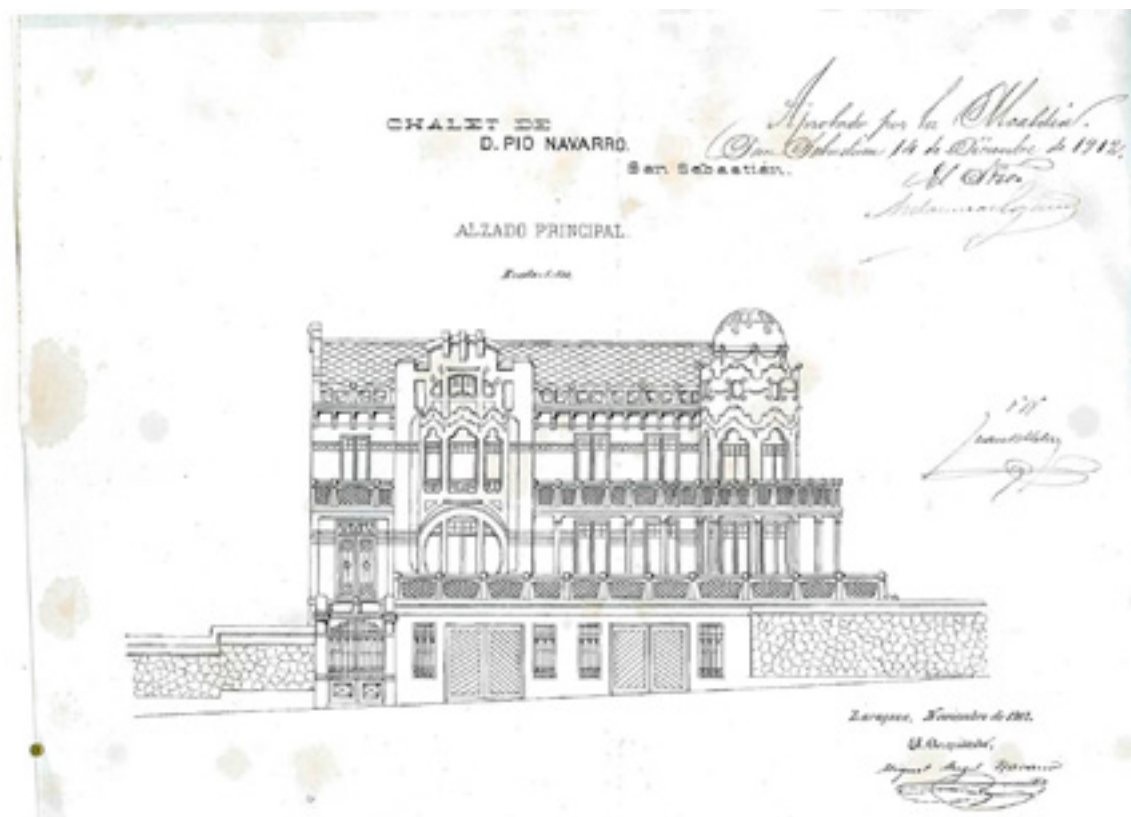
[ Figura 9. Alzado Principal del proyecto de Villa Pura, fechado en 1912 y firmado por el arquitecto Miguel Ángel Navarro Pérez. ] Fuente: Archivo Histórico Municipal de San Sebastián.
